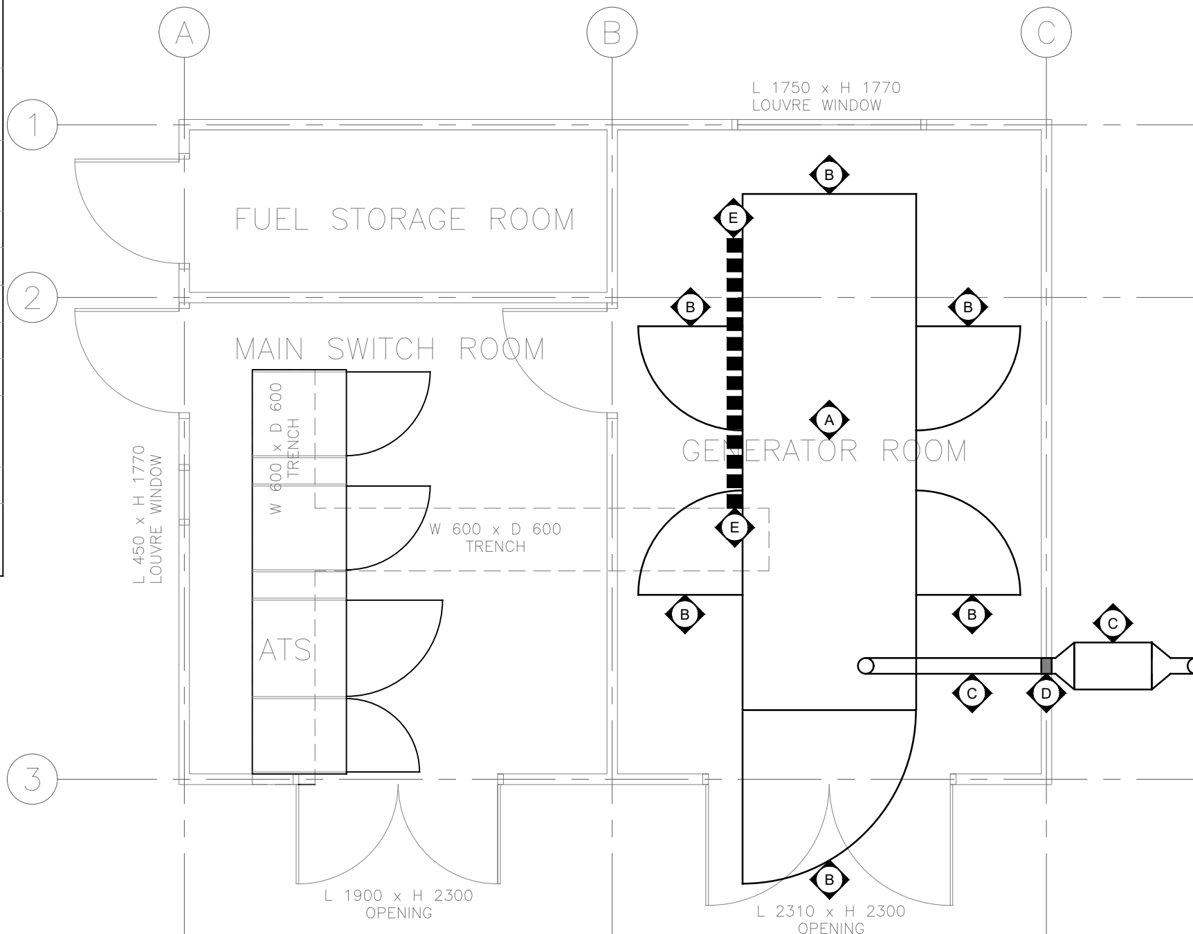
GENERATOR LAYOUT SCALE: 1:50 @ A3
